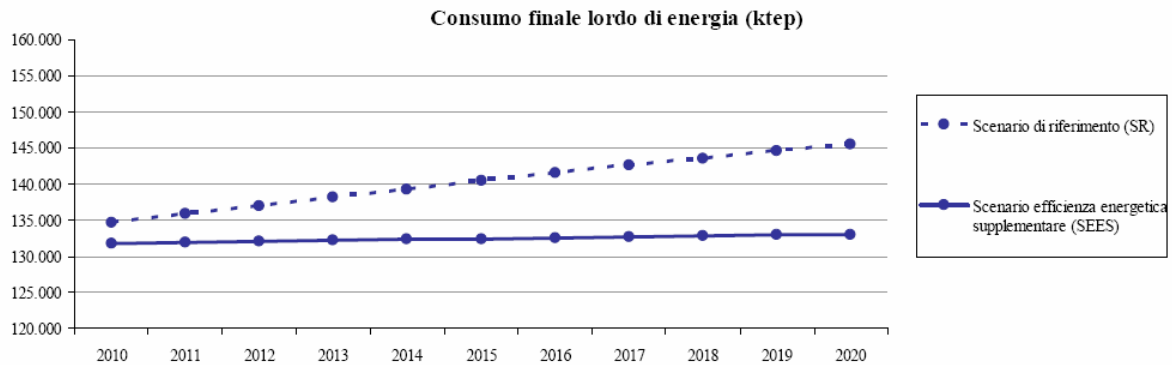
Fig. 1 – Stime (PAN) dell'evoluzione dei CFL al 2020 per l'Italia
