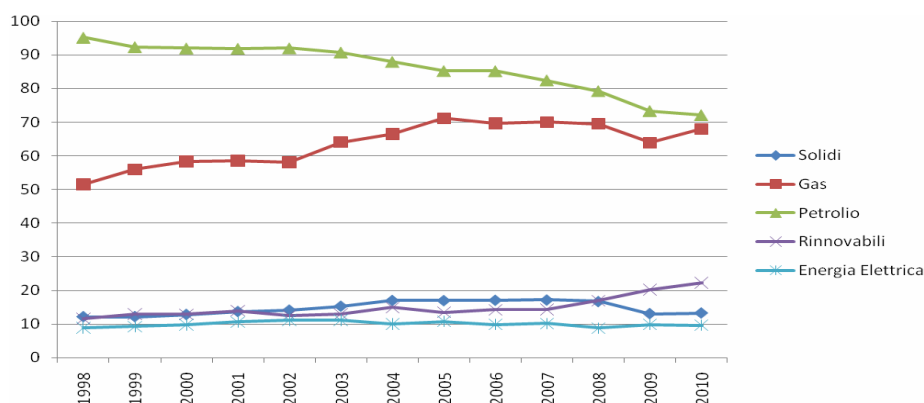
Fig. 3 - Domanda d'energia primaria (Mtep) per singola fonte in Italia (Fonte REA2009 5 )
