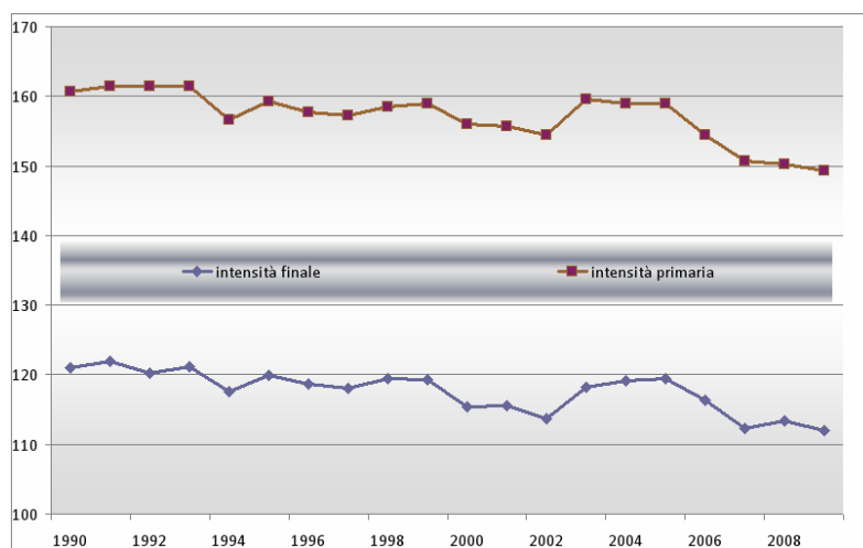
Fig. 2 - Intensità energetica dell'Italia (tep/M€ - Fonte ENEA)
